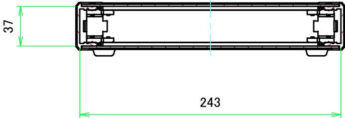
B-B ( 1 : 3.5 )
