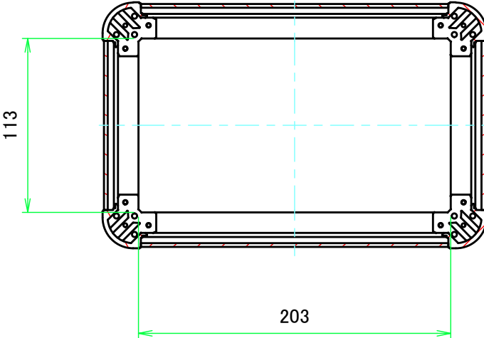
C-C ( 1 : 3.5 )
